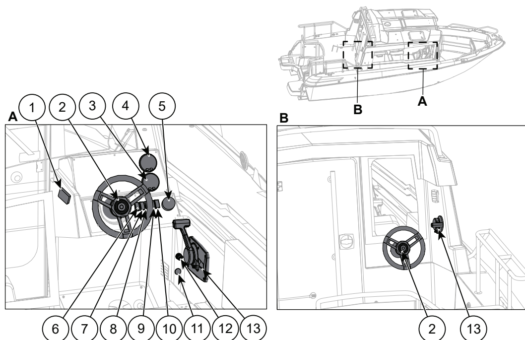
Figure 5.1 Commandes du poste de barre (A) et commandes optionnelles du poste de barre extérieur (B)
