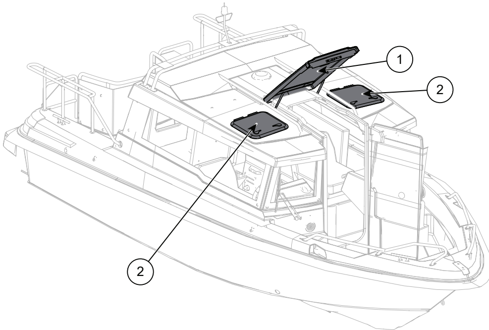
Figure 4.3 Cross 60 Cabin - Emplacement des panneaux de toit
