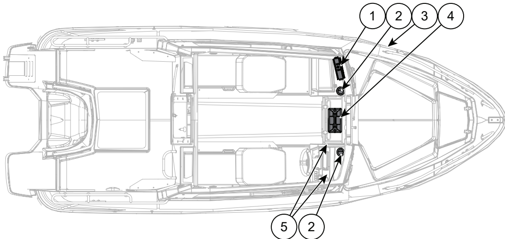
Figure 6.2 Cross 60 Cabin - Système de chauffage
