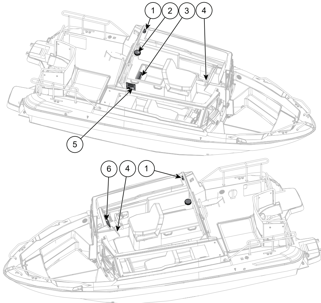
Figure 8.3 Cross 60 Cabin - Équipement électrique
