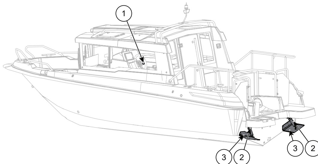
Figure 5.5 Cross 60 Cabin - Système de trim
