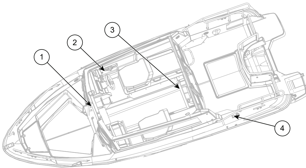
Figure 2.1 Cross 60 Cabin - Étiquettes de sécurité
