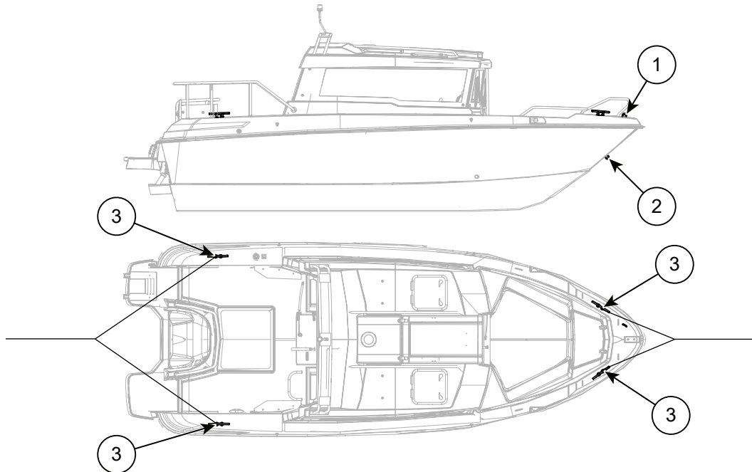
Figure 5.7 Cross 60 Cabin - Points d'amarrage et de remorquage
