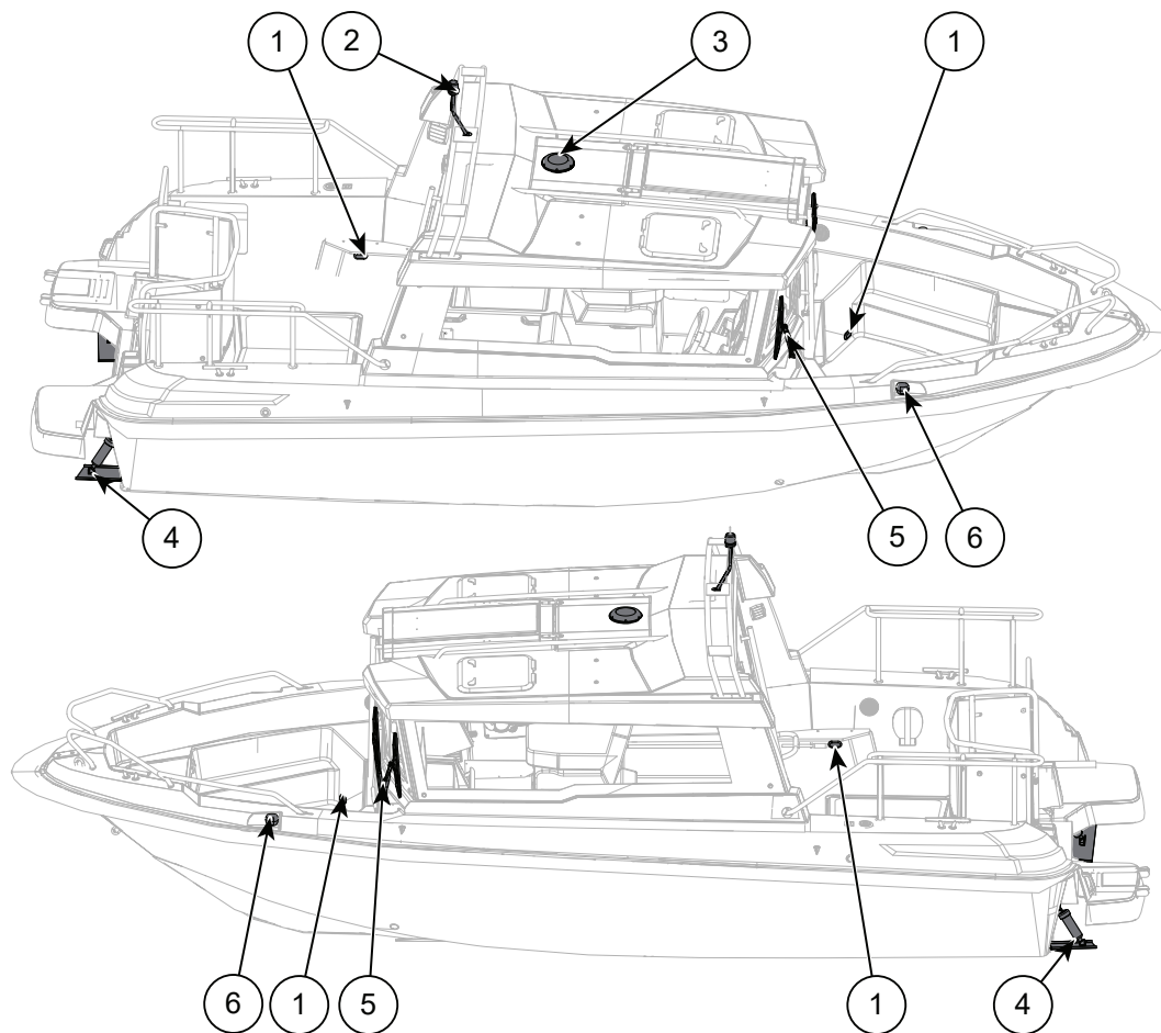
Figure 8.2 Cross 60 Cabin - Équipement électrique extérieur
