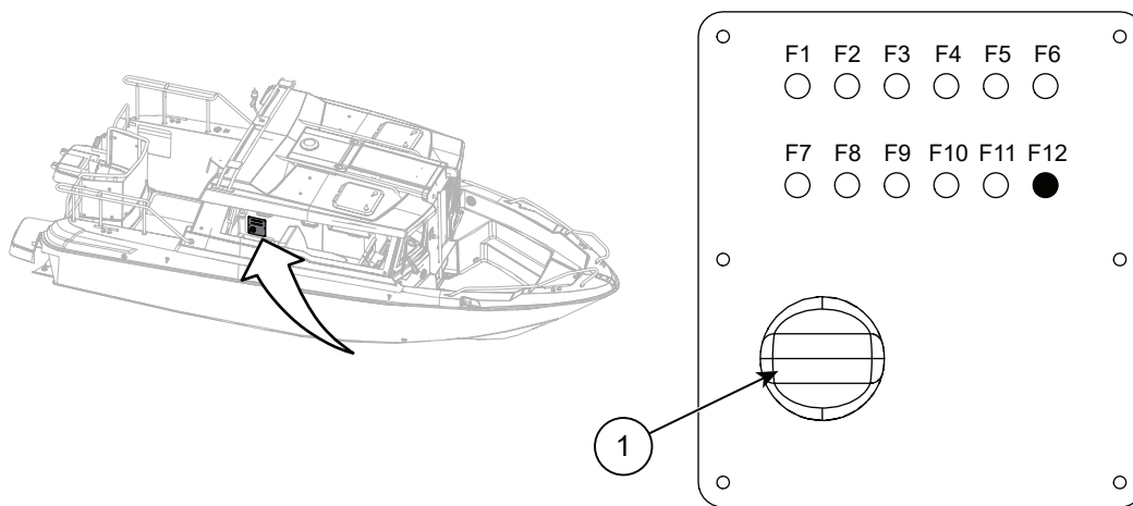
Figure 8.1 Cross 60 Cabin - Interrupteur principal et panneau de fusibles
