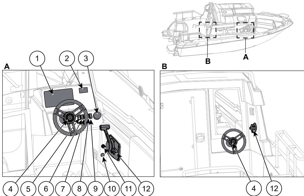
Figure 5.2 Commandes du poste de barre (A) avec Cross Q et commandes optionnelles du poste de barre extérieur (B)
