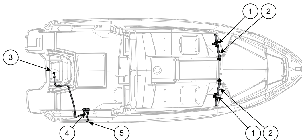
Figure 9.1 Cross 60 - Dispositif de vidange de la cabine
